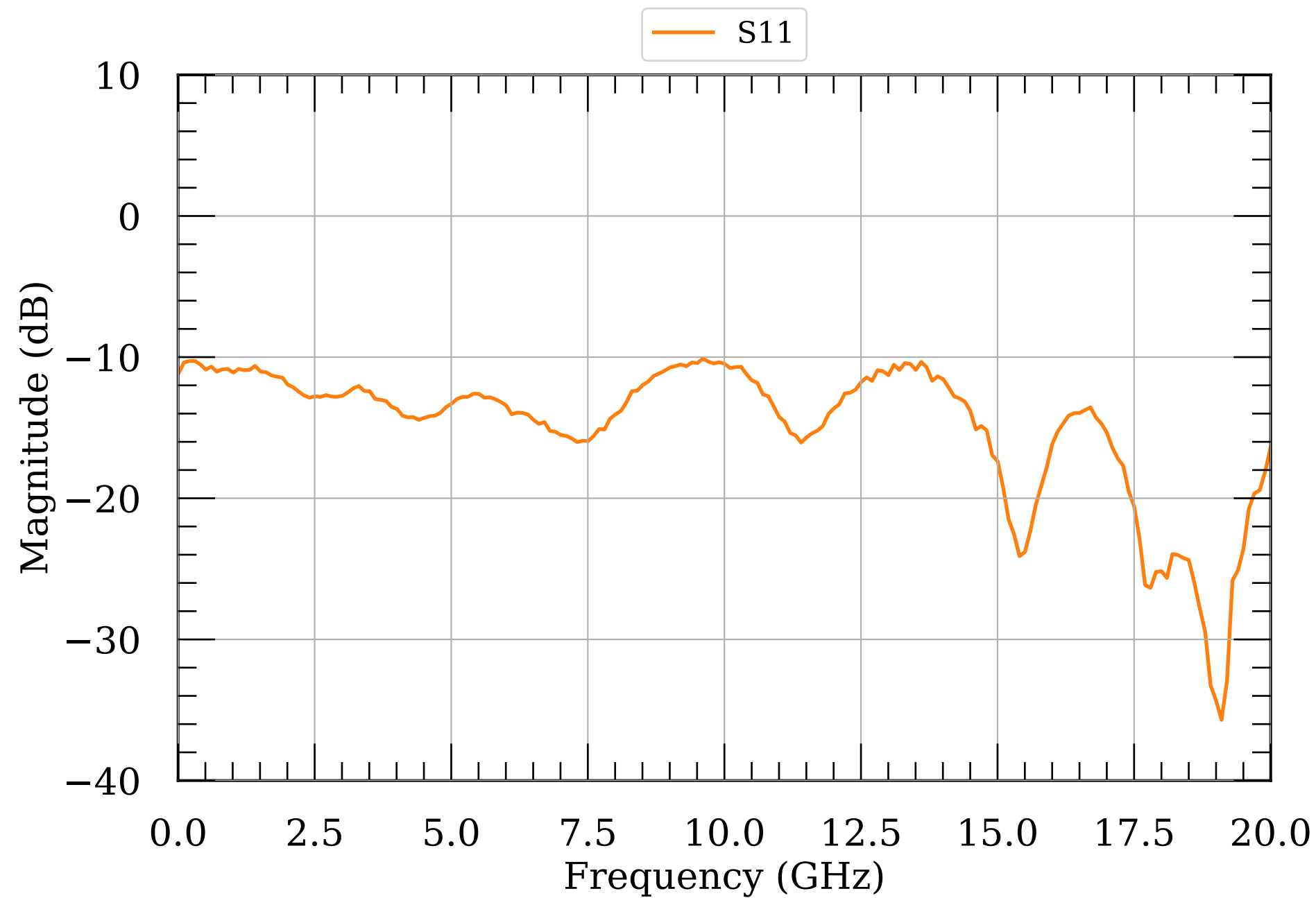
LNA S-params module070
